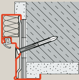
Diagonalbefestigung (Mauerwerk)
