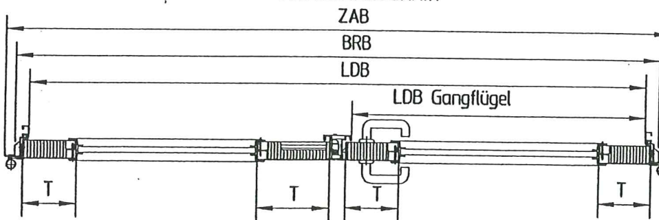
Horizontalschnitt
